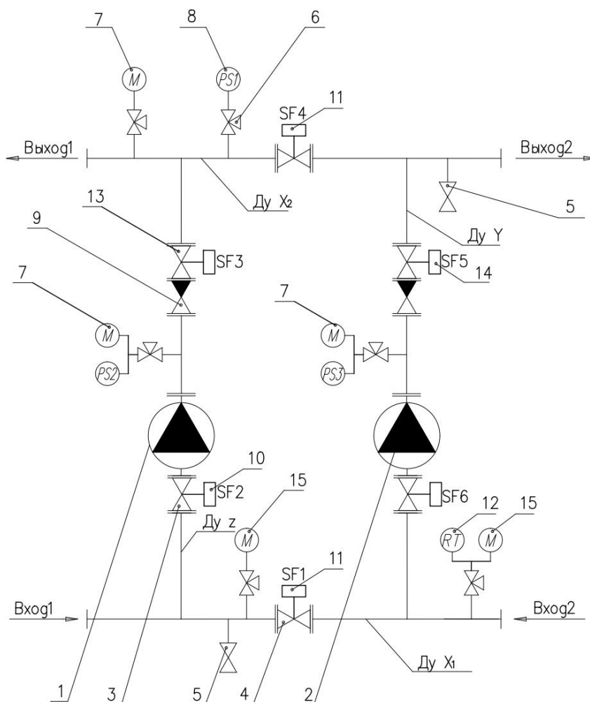
Гидравлическая схема насосной установки «Спрут-НС» для двух пожарных насосных агрегатов.
