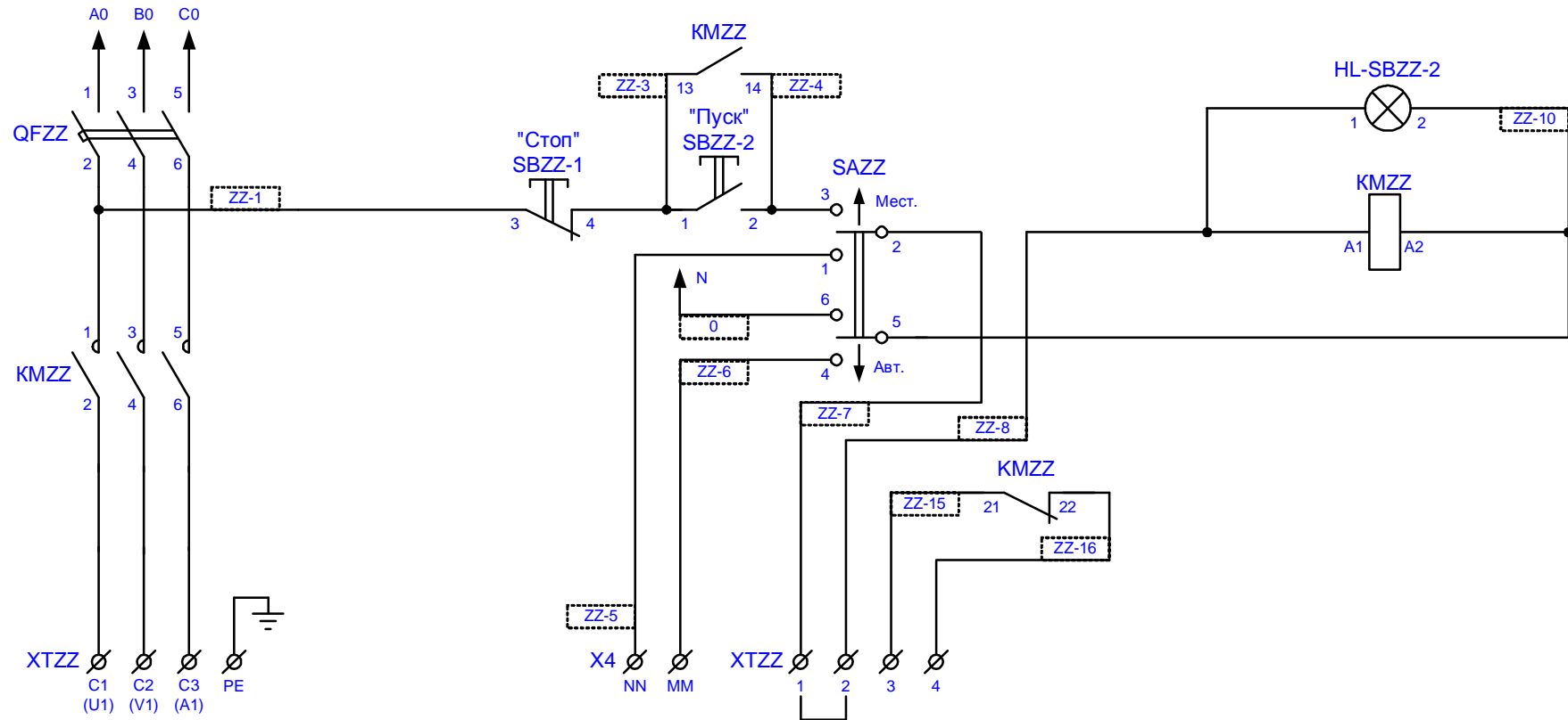
Схема управления пожарным насосом. Пример: ПН/15/3/0
